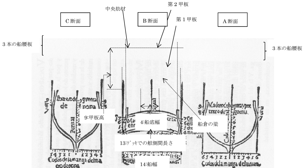
ガルシア・デ・パラシオ「150 トネラーダの船の断面図」
