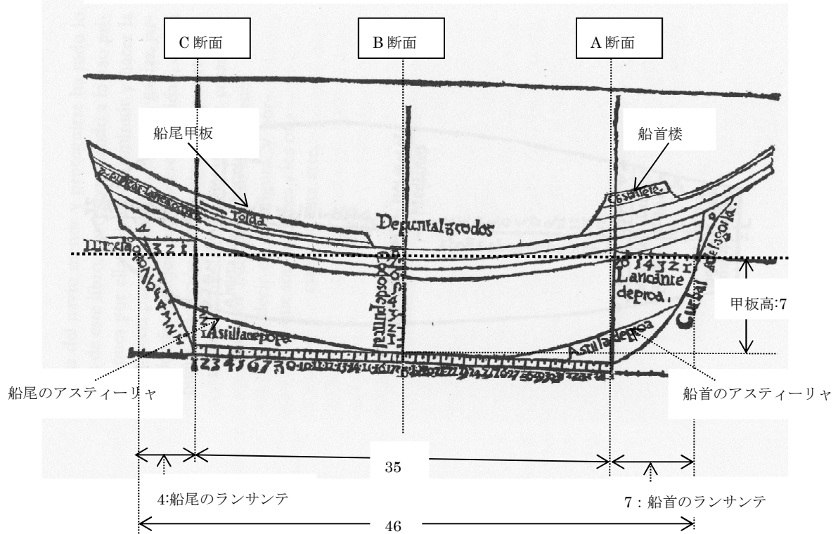
ガルシア・デ・パラシオ「150 トネラーダの船の側面図」 (単位：コード)
